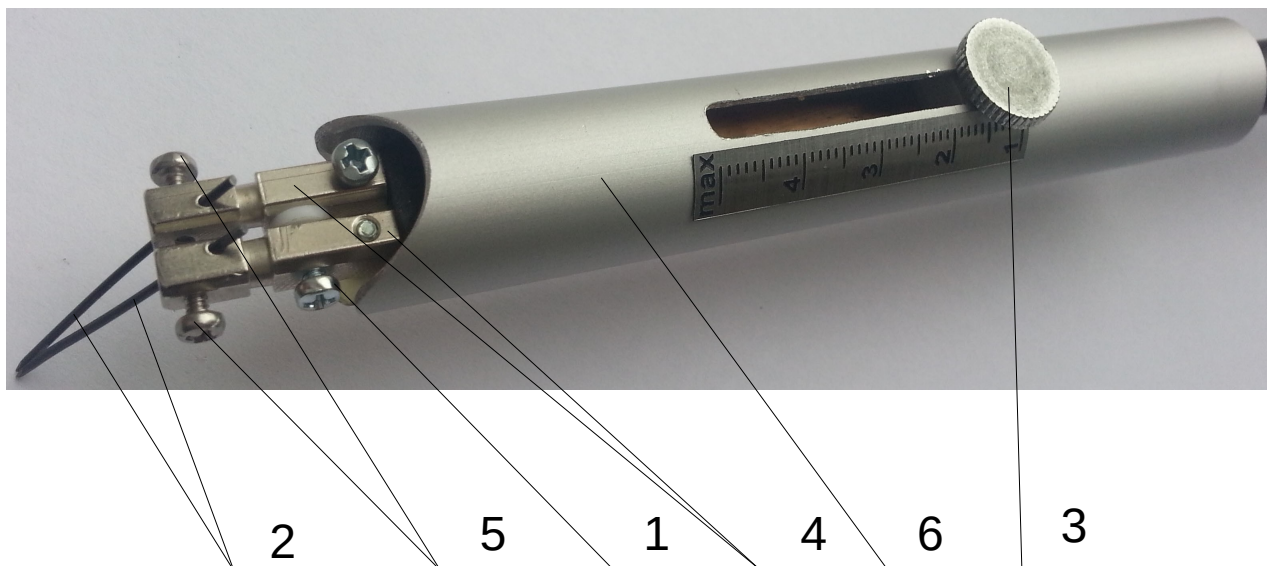
Рис. 1. Инструмент с установленным сдвоенным электродом.
