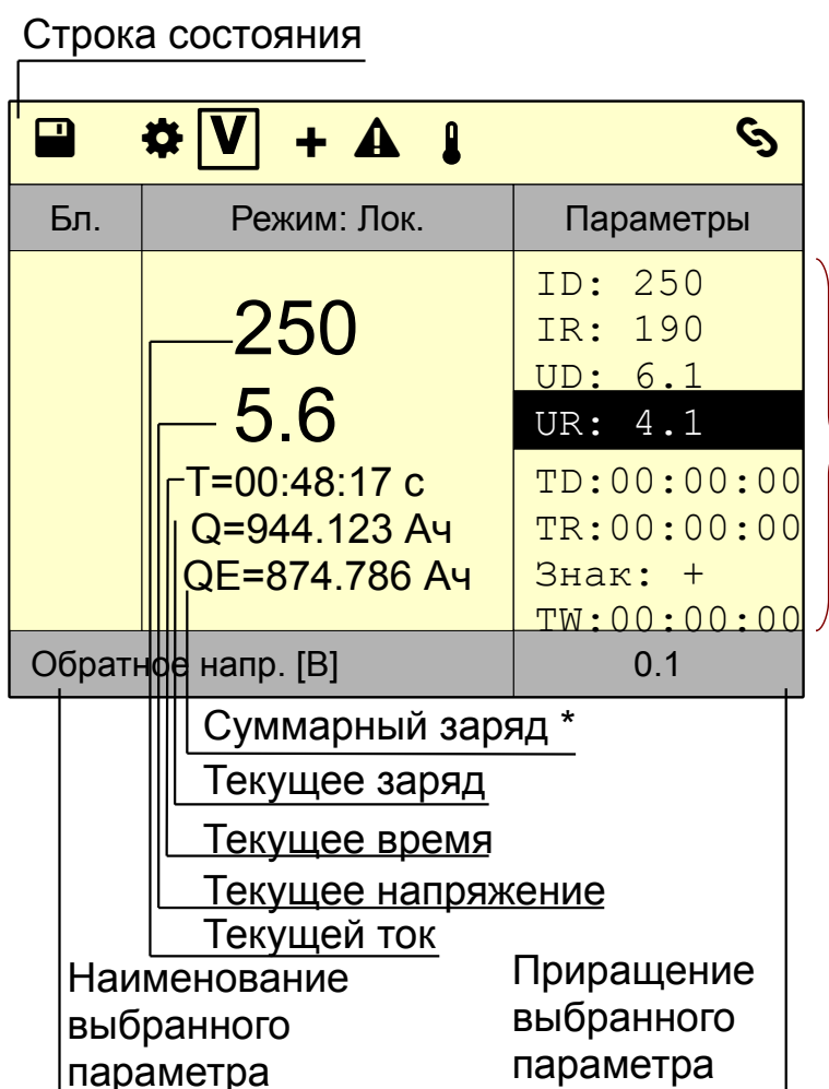
Рис. 4. Вид ЖК дисплея в режиме «ЛОКАЛЬНЫЙ»
